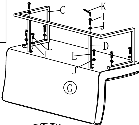
M6X15 Ⓛ X6
